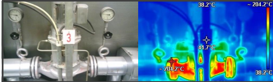
Aufnahme einer Wärmebildkamera zur Überprüfung des Abwärmepotentials
